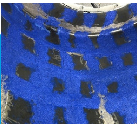
Turboseparator w zakładzie recyklingu Belzona 1818
